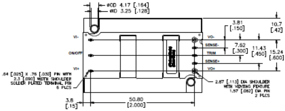
Bottom View*
